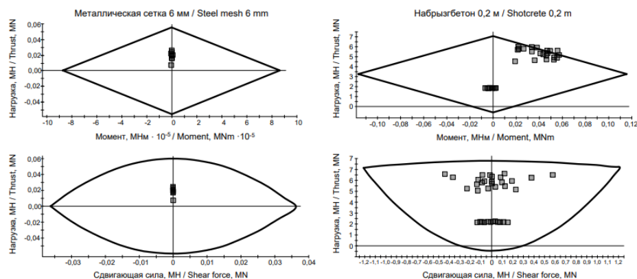
Рис. 3. Паспорт несущей способности набрызгбетонной крепи, армированной металлической сеткой/
