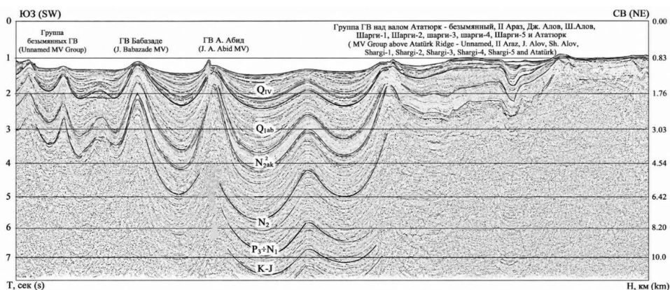
Рис. 8. Временной разрез через группу ГВ над вало Атаюрк / Fig. 8. Time section through a group of mud volcanoes (MV) over the Ataturk Rise
