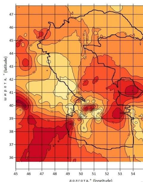
Рис. 2. Карта теплового потока ( \text{мВт/м}^2 ) Каспийского региона / Fig. 2. Heat flow map ( \text{mW/m}^2 ) of the Caspian region
