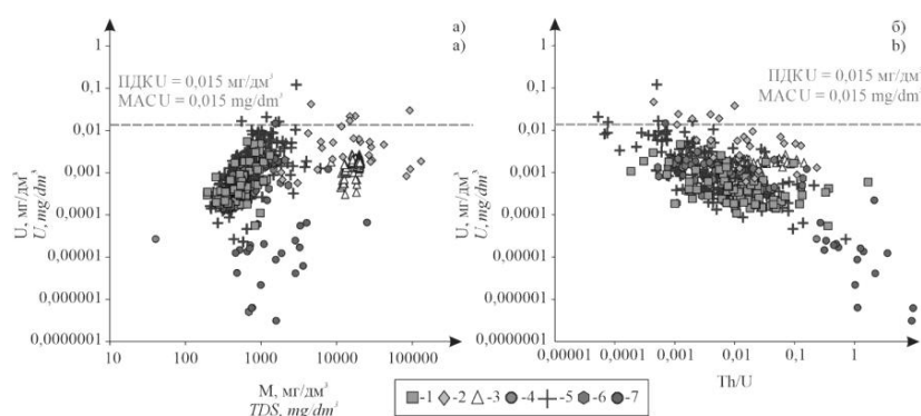
Рис. 4. Зависимость содержания урана в природных водах Крымского полуострова от величины их общей минерализации (а) и отношения \text{Th/U} (б).
